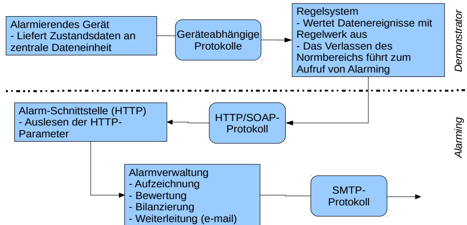
Abbildung 4: Nachrichtenfluss am fortiss Demonstrator
